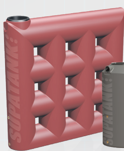
1000S Slimline W. 360 L. 1895 H. 1795
