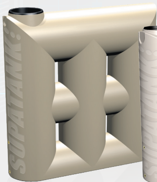
2000SK Slimline W. 680 L. 2000 H. 2180
