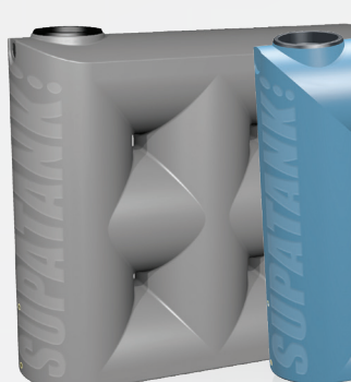
3000S Slimline W. 780 L. 2390 H. 2180
