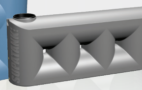
2000SS Slimline W. 770 L. 1560 H. 2150
