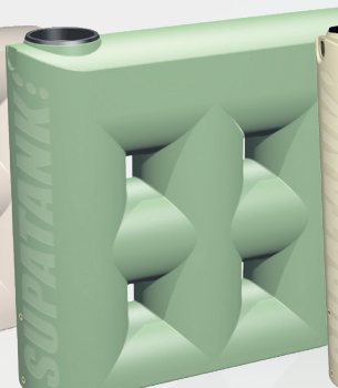
2300S Slimline W. 650 L. 2230 H. 2100
